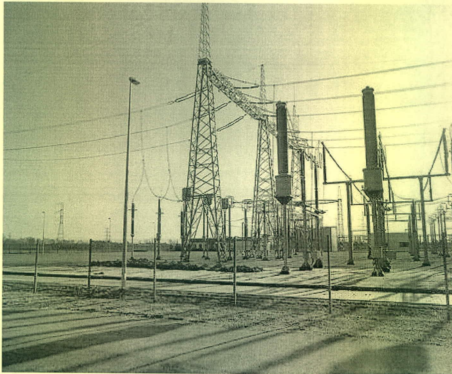
Hình ảnh Đường dây và trạm biến áp 110 kV Tân Tạo
